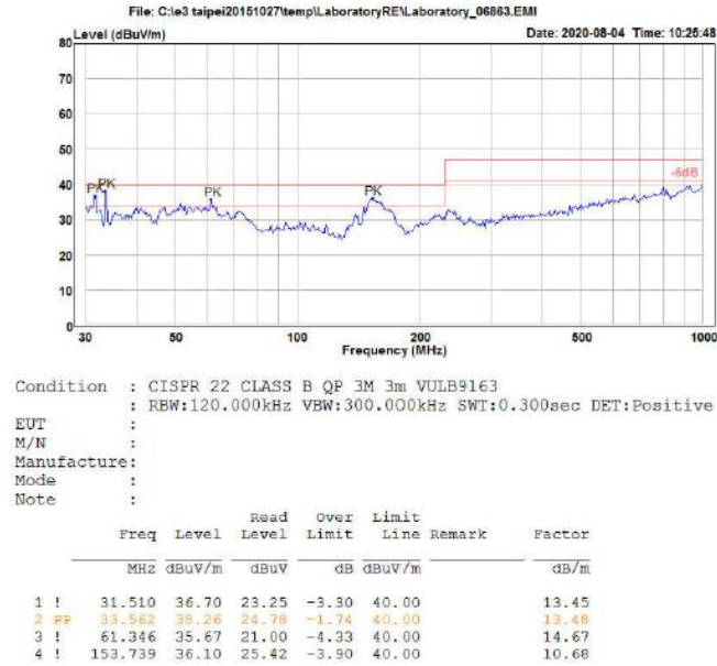
图 3-7 辐射测试垂直方向
