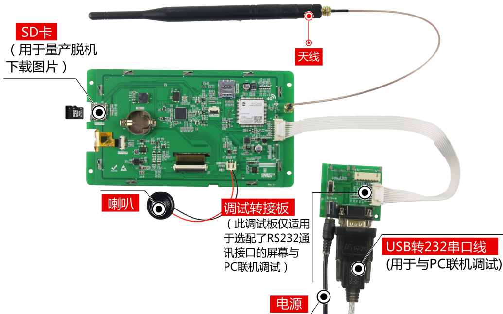
图 1-5 调试工具图
