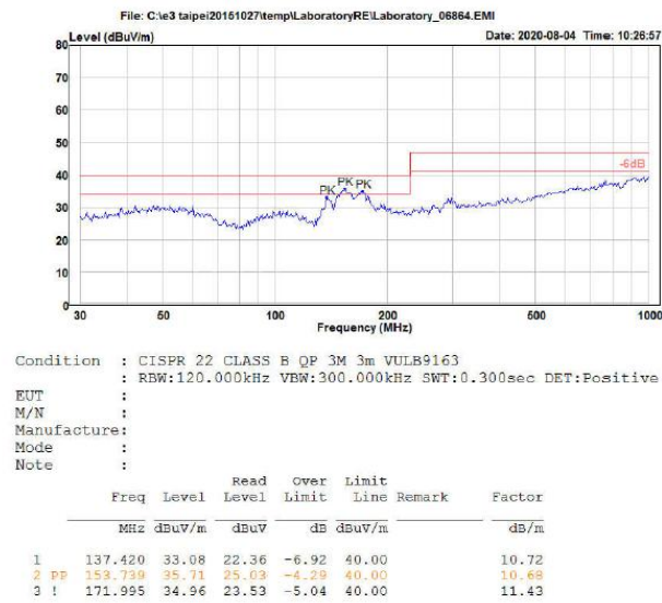
图 3-6 辐射测试水平方向
