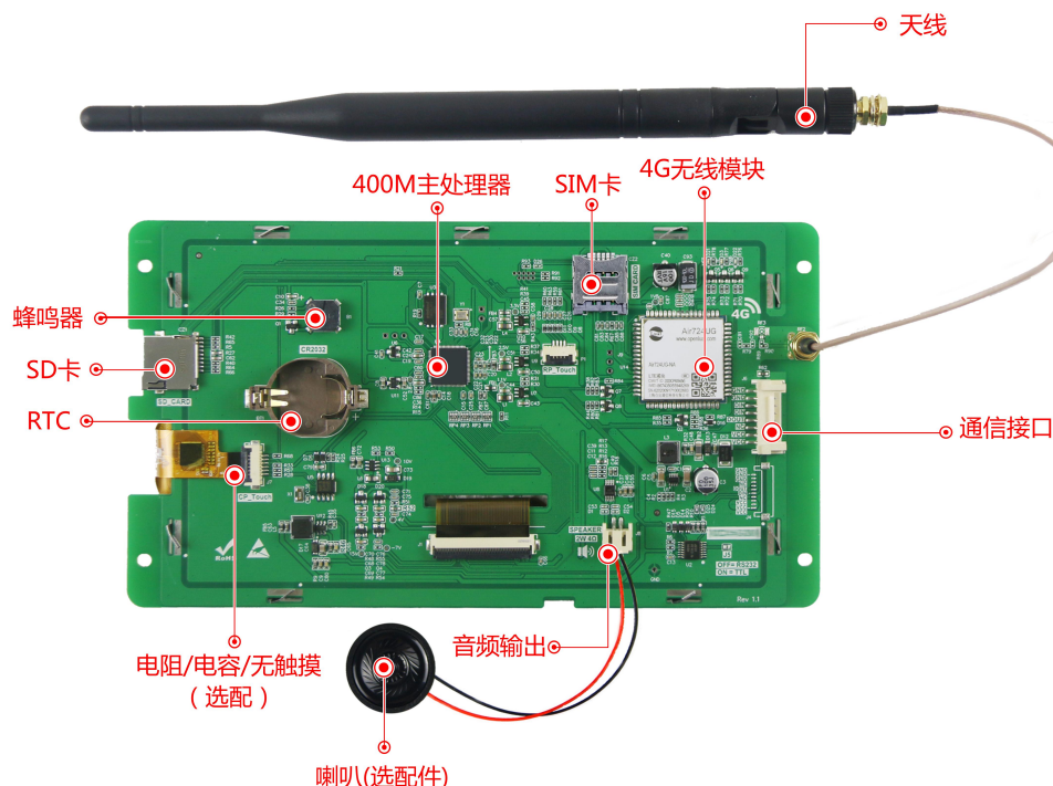
图 1-4 硬件配置图
